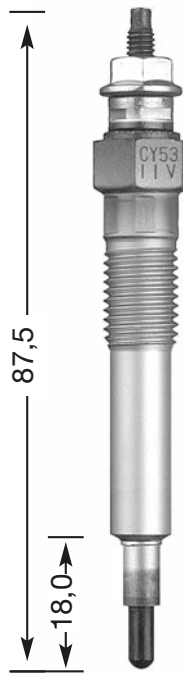
CY 53 † M 10 x 1.25 12 Hex 11 V
