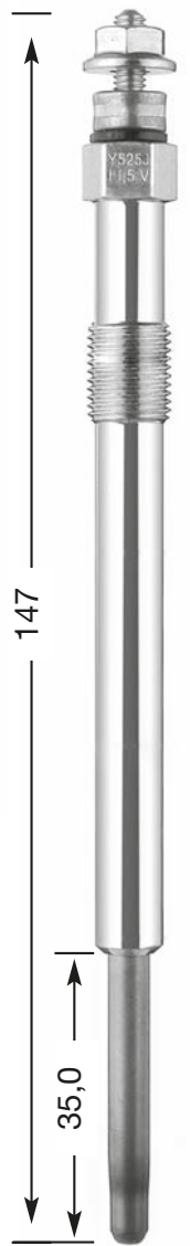
Y-525 J M 10 x 1.0 10 Hex 11,5 V DP 35
