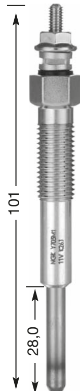
Y-703 M1 M 10 x 1.25 12 Hex 11 V
