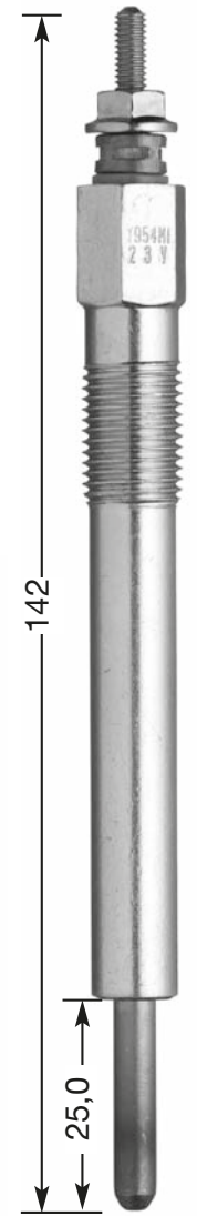
Y-954 M1 M 12 x 1.25 12 Hex 23 V
