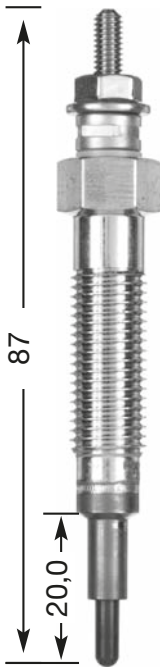
CZ 256 M 10 x 1.25 12 Hex 11 V
