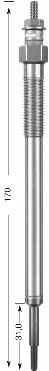
CZ 251 M 10 x 1.25 12 Hex 11 V DP 76
