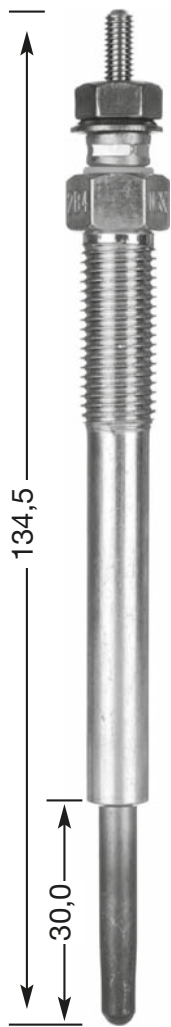
Y-527 J M 10 x 1.25 12 Hex 11 V DP 67
