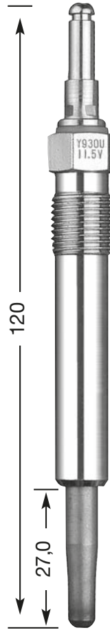
Y-930 U M 12 x 1.25 12 Hex 11,5 V DP 30
