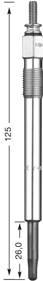
Y-729 U M 10 x 1.0 10 Hex 11,5 V DP 34
