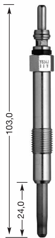
Y-534 J M 10 x 1.25 10 Hex 11 V DP 36
