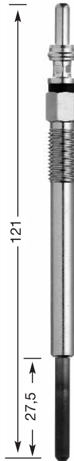
YE 06 M 8 x 1.0 8 Hex 11 V
